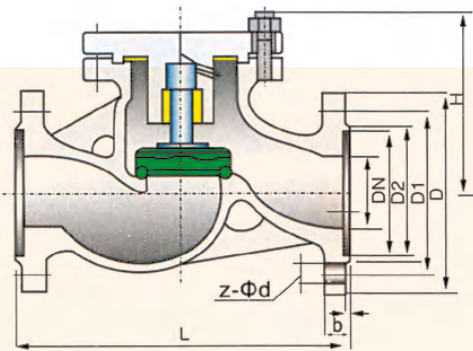
H41W升降式止回阀
